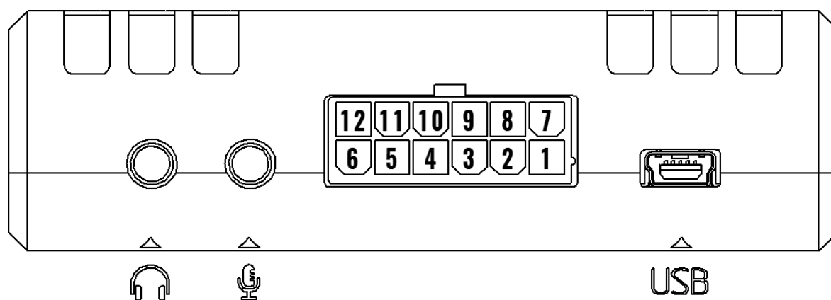
Рисунок 2.2 Нумерация выводов терминала
