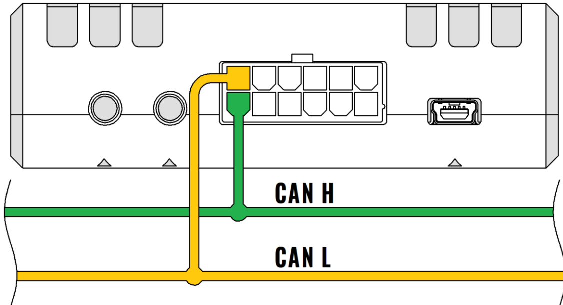
Рисунок 2.18 Подключение к шине CAN
