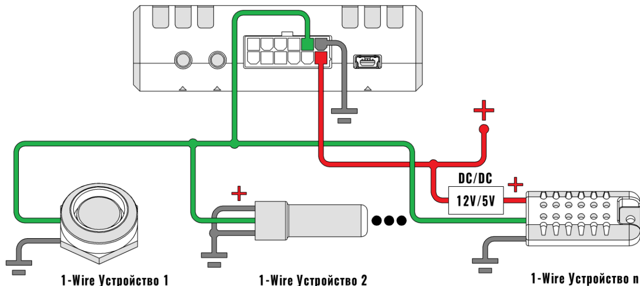
Рисунок 2.20 Подключение устройств по 1-Wire
