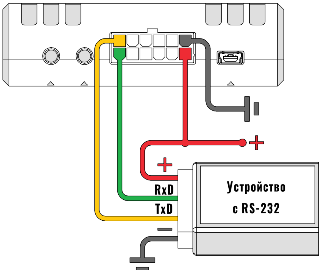
Рисунок 2.19 Подключение по интерфейсу RS-232
