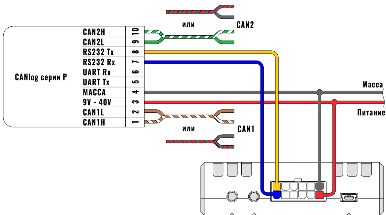
Рисунок 2.21 Подключение CAN-LOG по RS-232
