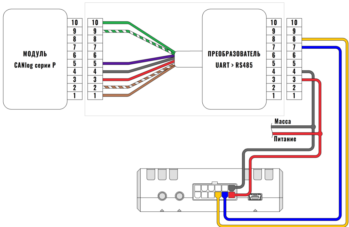
Рисунок 2.22 Подключение CAN-LOG через переходник UART-RS485
