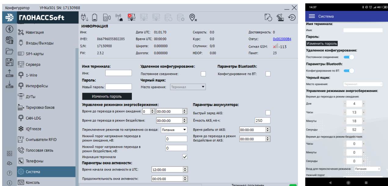
Рисунок 3.35 Вкладка «Система»
