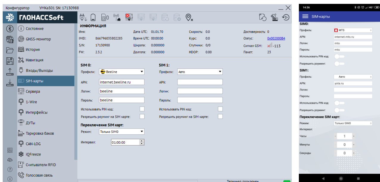
Рисунок 3.20 Вкладка «SIM-карты»
