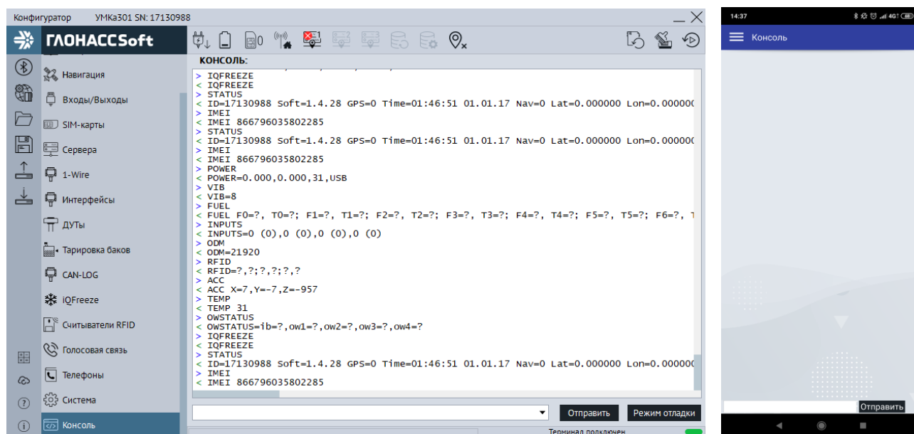
Рисунок 3.36 Вкладка «Консоль»
