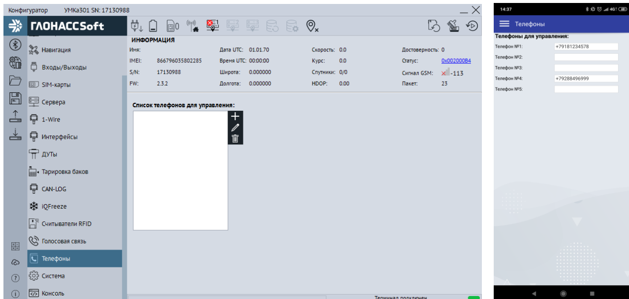
Рисунок 3.32 Вкладка «Телефоны»
