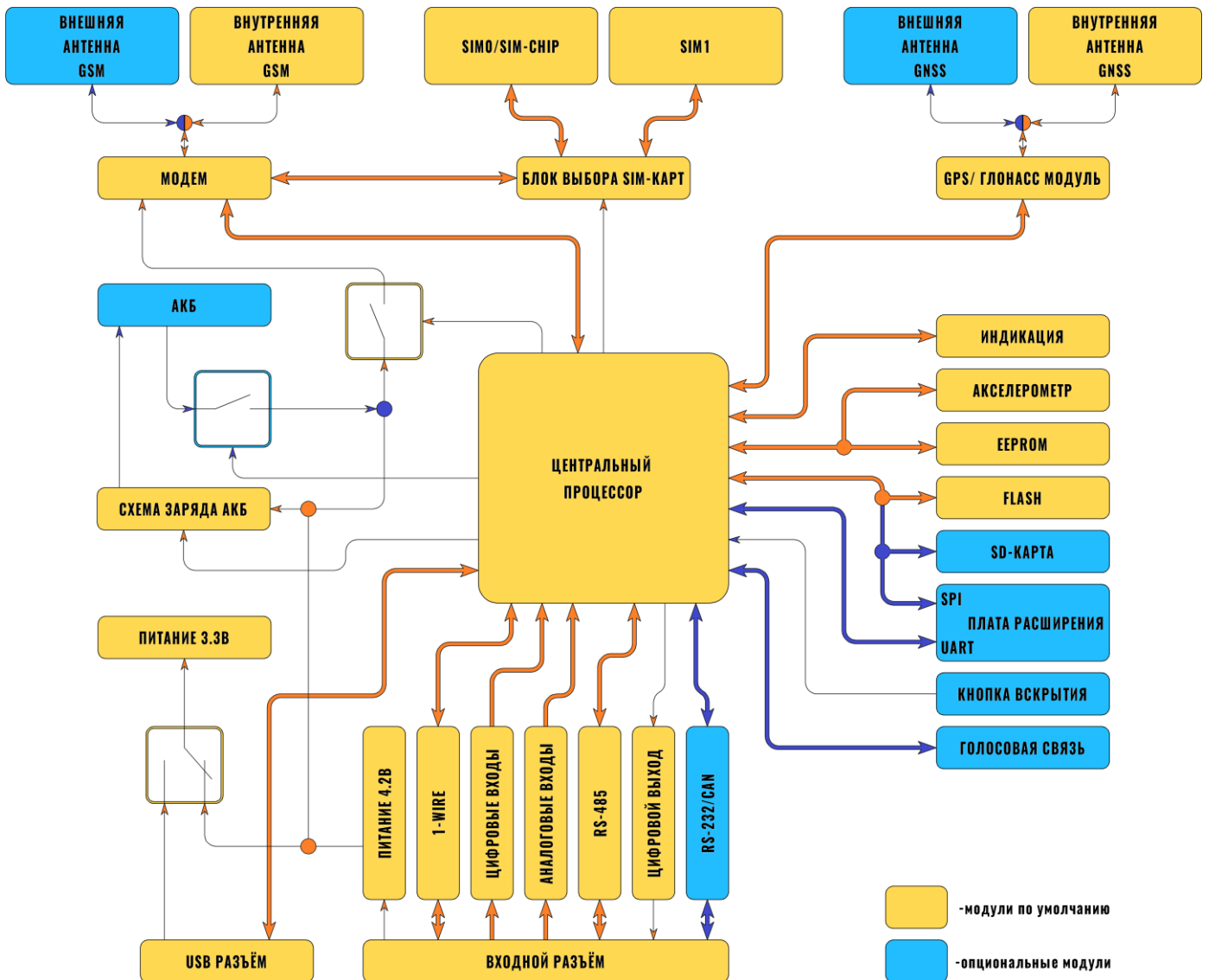
Рисунок 1.3 Блок-схема навигационного терминала
