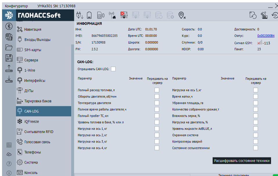
Рисунок 3.27 Вкладка «CAN-LOG»
