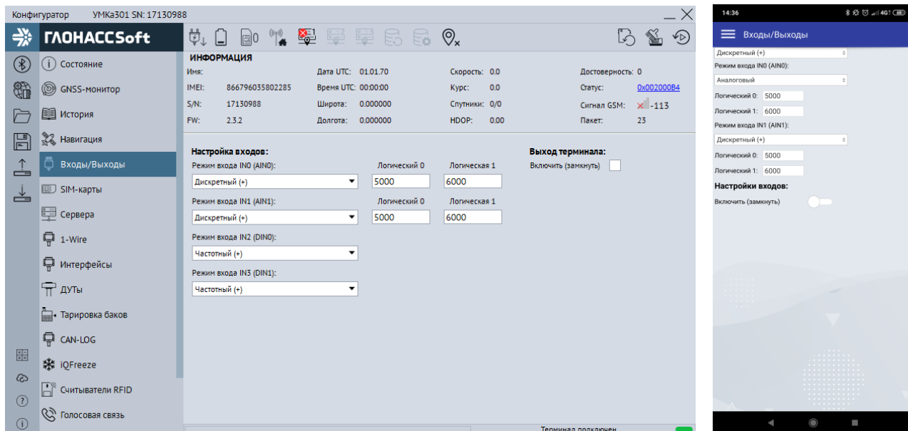
Рисунок 3.19 Вкладка «Входы/Выходы»
