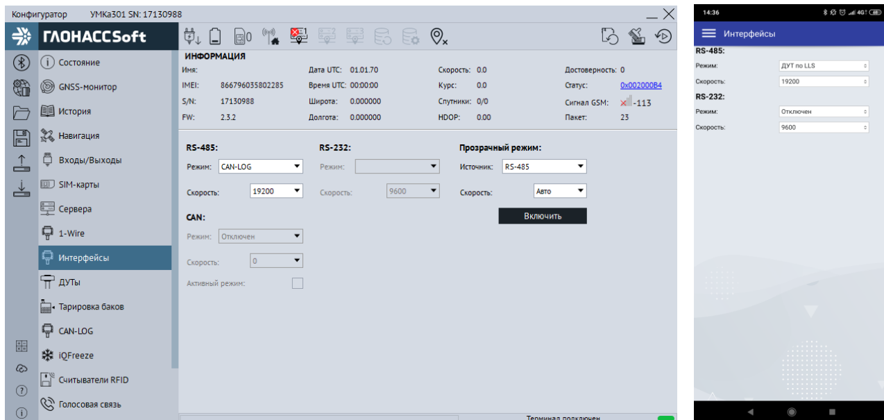
Рисунок 3.23 Вкладка «Интерфейсы»
