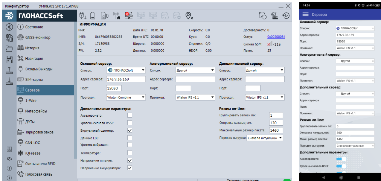
Рисунок 3.21 Вкладка «Сервера»
