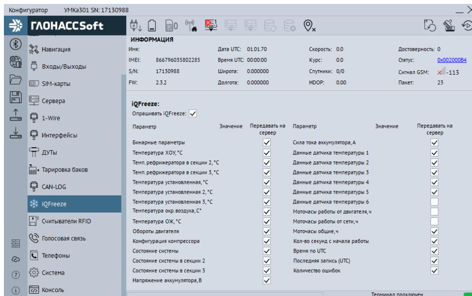
Рисунок 3.29 Вкладка «iQFreeze»
