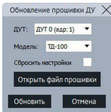
Рисунок 3.26 Обновление ДУТ
