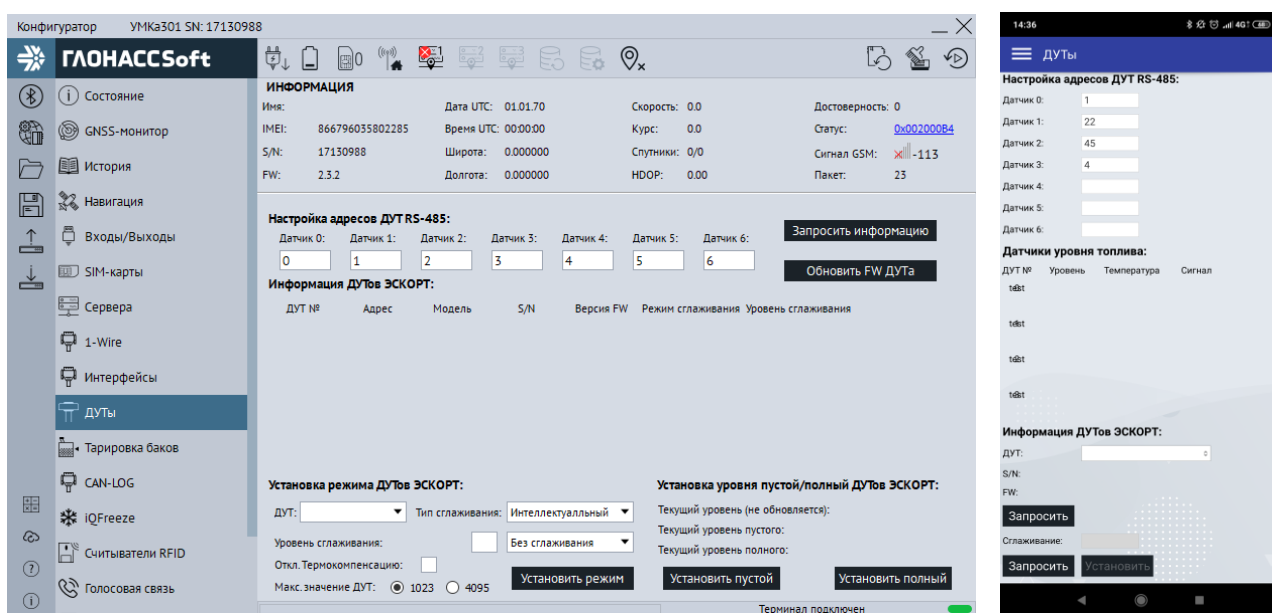
Рисунок 3.25 Вкладка «ДУТы»
