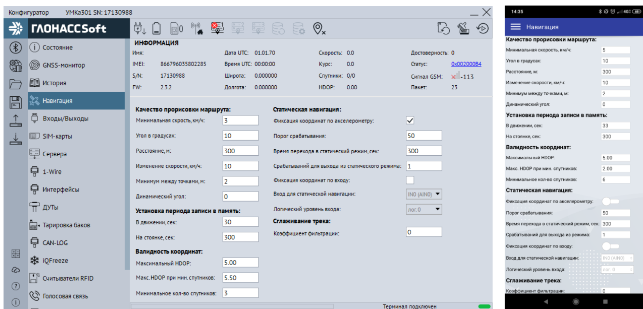
Рисунок 3.17 Вкладка «Навигация»
