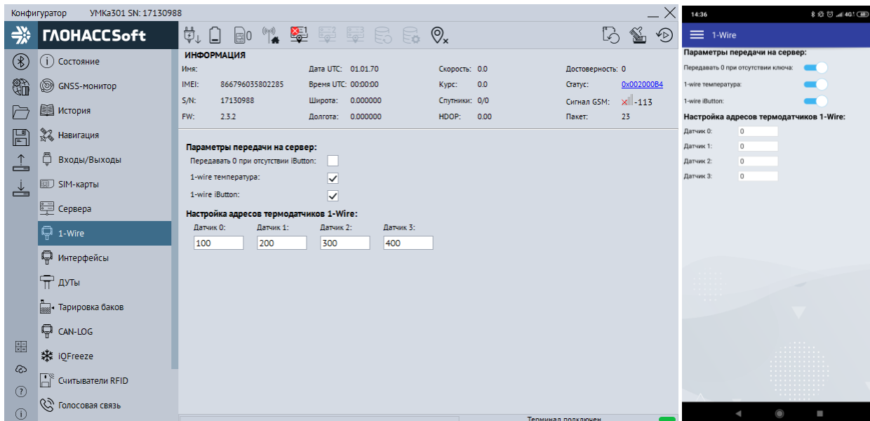
Рисунок 3.22 Вкладка «1-Wire»
