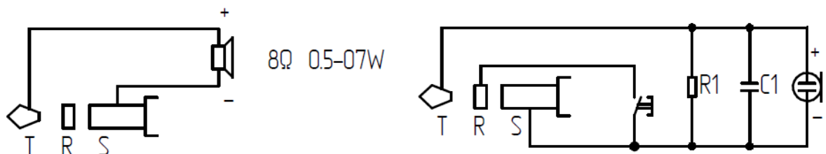
Рисунок 2.23 Схема распайки тангенты
